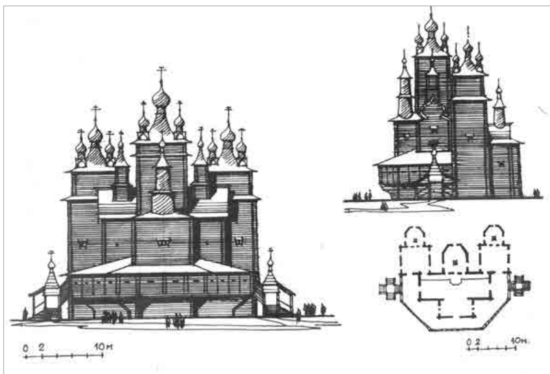
Ил. 12. Воскресенский собор. 1682 – 1684 гг. Западный и южный фасады. Реконструктивный рисунок Ю. С. Ушакова
